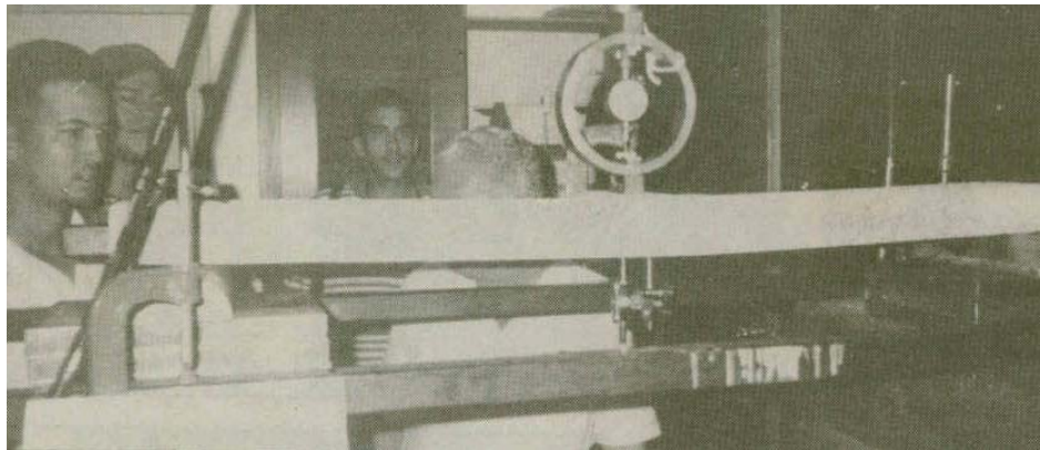
Desarrollo de fisuras en la viga de hormigón previo a su falla.
